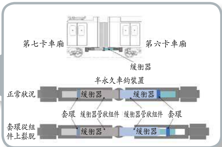
港鐵以圖解釋車鈎內緩衝器套環鬆脫。
